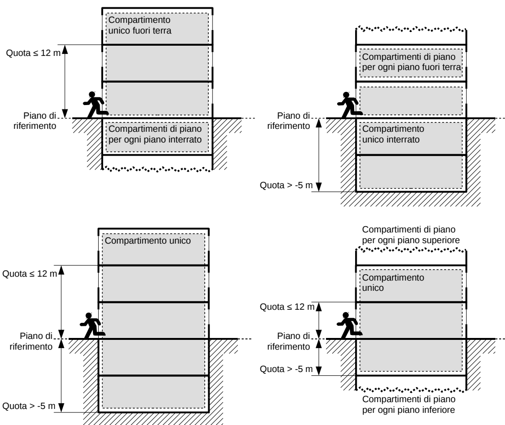
Illustrazione 6-1: Esempi di compartimentazione multipiano
